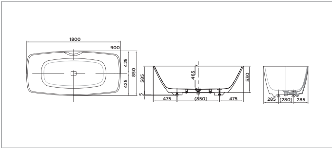
PJY1804HPWE PJY1804HPWE Bồn tắm GAGALATO đặt sàn
