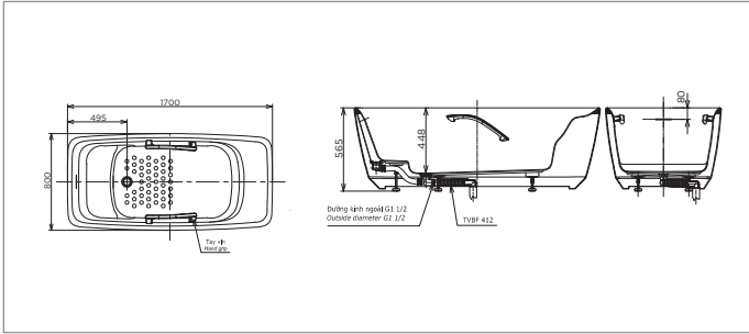
PJY1724HPWE PJY1724PWE PJY1724HPWE Bồn tắm GAGALATO đặt sàn Bao gồm tay vịn Không bao gồm tay vịn
