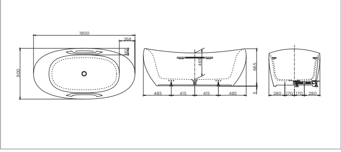
PJY1814HPWE PJY1814HPWE Bồn tắm GAGALATO đặt sàn, xả nhấn Bao gồm tay vịn
