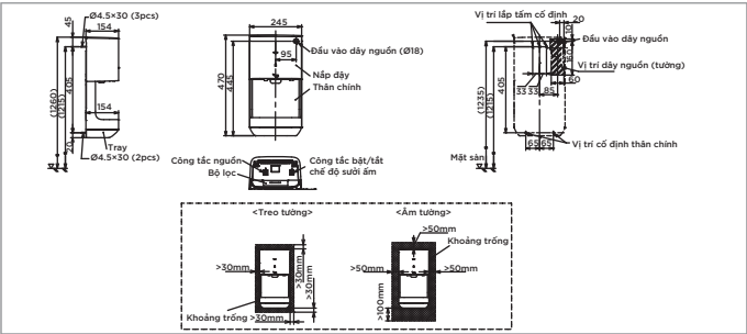
TYC322W TYC322W Máy sấy tay
