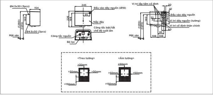
TYC322WF TYC122W TYC322WF TYC122W Máy sấy tay
