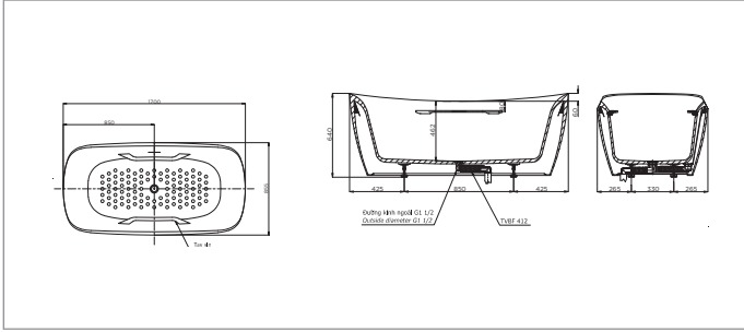
PJY1734HPWE PJY1734PWE PJY1734HPWE Bồn tắm GAGALATO đặt sàn Bao gồm tay vịn Không bao gồm tay vịn
