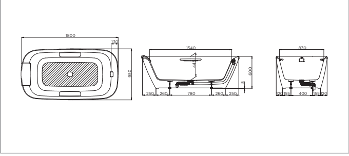
PJY1886HPWMNE PJY1886HPWMGE PJY1886HPWMNE Bồn tắm GAGALATO đặt sàn, xả nhấn Bao gồm tay vịn
