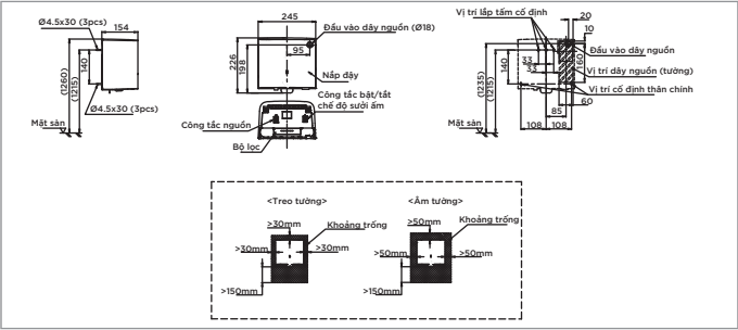
TYC322M TYC322M Máy sấy tay
