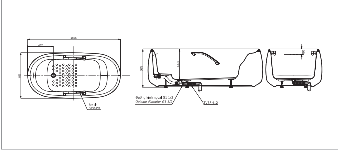
PJY1744HPWE PJY1744PWE PJY1744HPWE Bồn tắm GAGALATO đặt sàn bao gồm tay vịn PJY1744PWE Không bao gồm tay vịn
