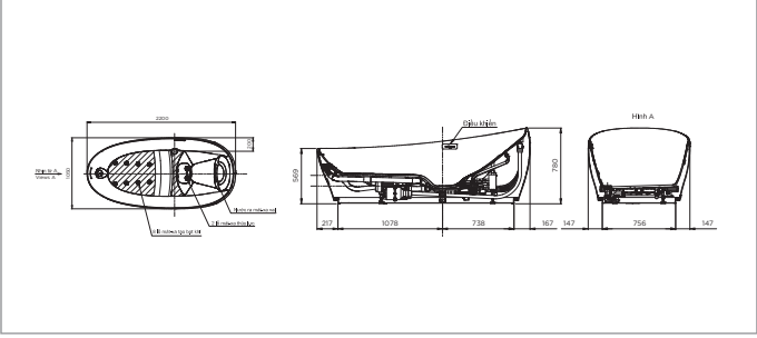
PJYD2200PWE PJYD2200PWE Bồn tắm nổi đặt sàn
