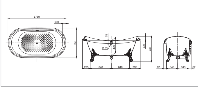
FBY1756PTGE FBY1756PTNE FBY1756PTGE Bồn tắm đặt sàn gang trắng men, chân mạ vàng FBY1756PTNE Bồn tắm đặt sàn gang trắng men, chân mạ bạc
